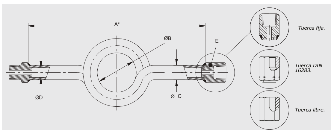
Fig 3. Dimensiones modelo 091.
